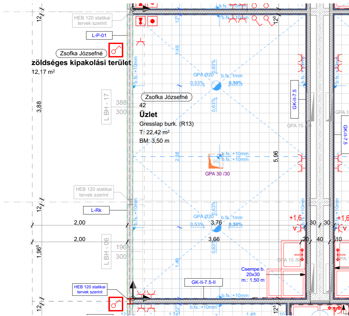
Bérlői földszinti alaprajz
