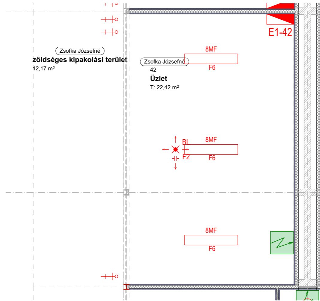
Bérlői állmenyezeti terv
